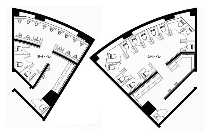
1F〔東側〕男女トイレ 図面
