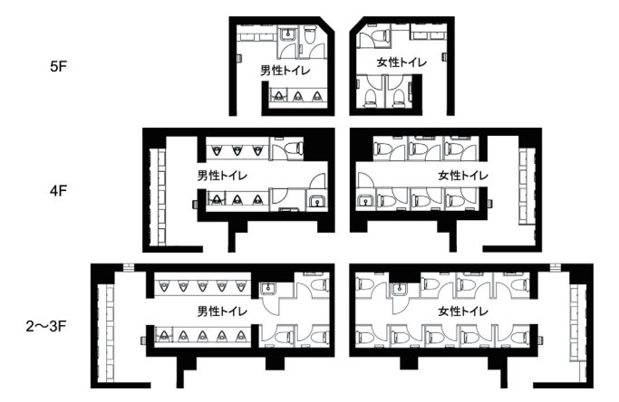
2～5F 男女トイレ図面
