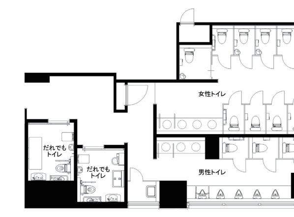
2Fトイレ図面
