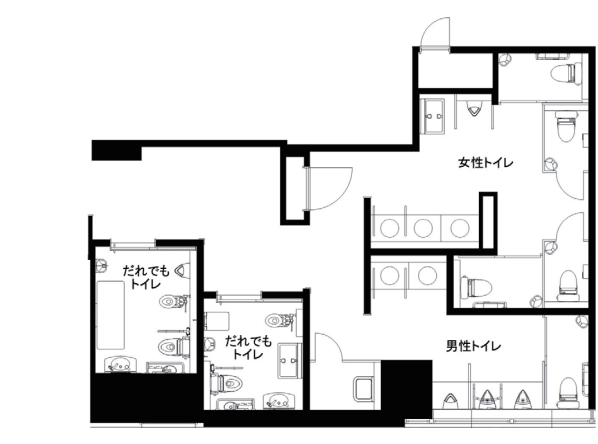
5Fトイレ図面
