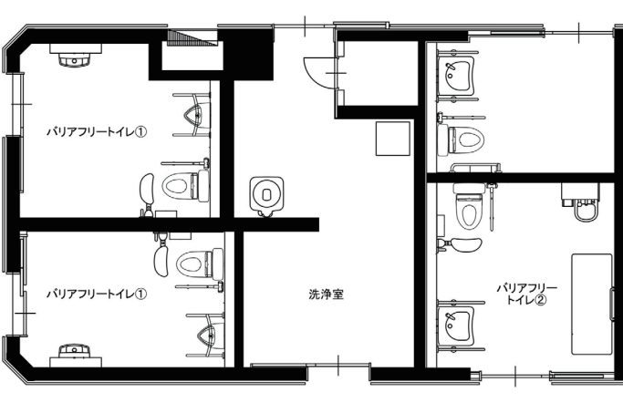
2F病棟 バリアフリースイレ図面
