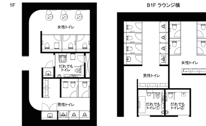
トイレ図面
